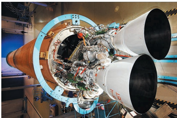
Ракетный двигатель РД-180
