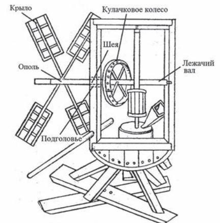
Рис. 3. Механизм ветряной мельницы, XVII в.
