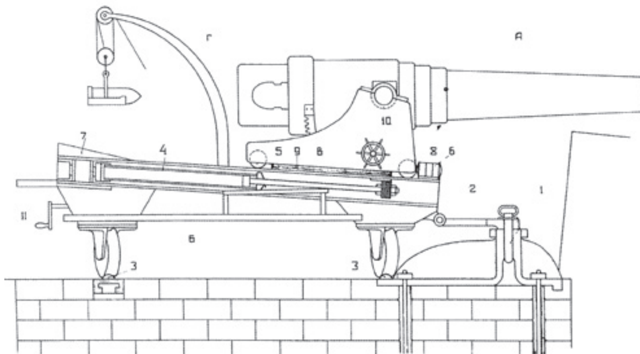
Лафет Семёнова для 11-дюймовой пушки обр. 1867 г. для стрельбы под углами возвышения 15^\circ .
