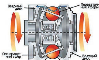
Втулка NuVinci
