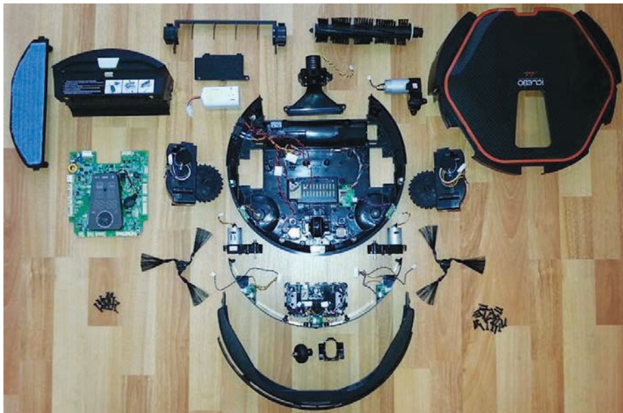
Современный робот-пылесос устроен довольно сложно. Когда он разобран, это видно наглядно
