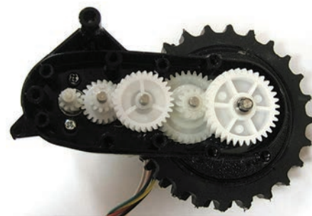
Вид редуктора одного из ведущих колёс
