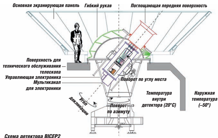
Схема детектора BICEP2
