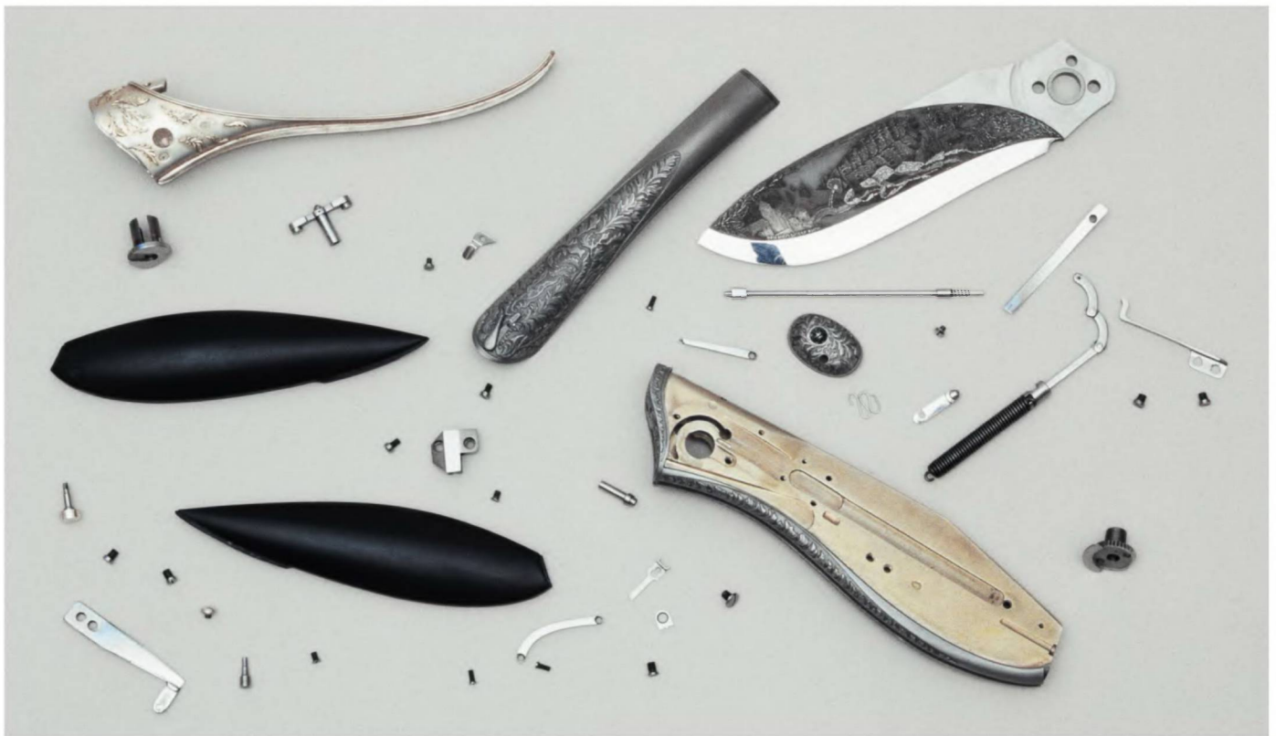
Полная разборка складного ножа «Блоха»
