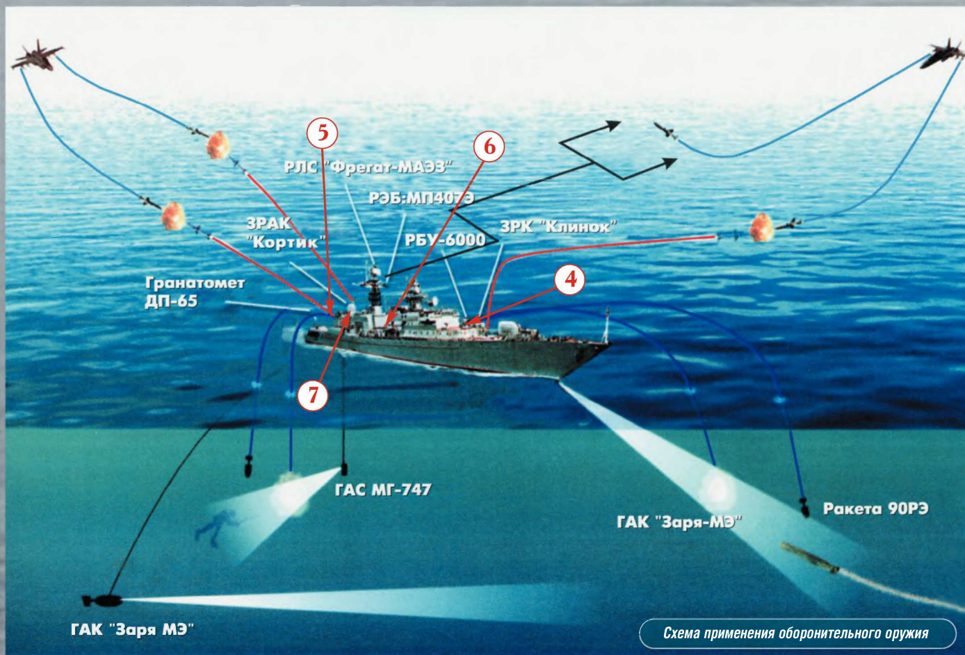
Зенитный ракетно-артиллерийский комплекс «Кортик». Он предназначен для уничтожения противокорабельных ракет противника
