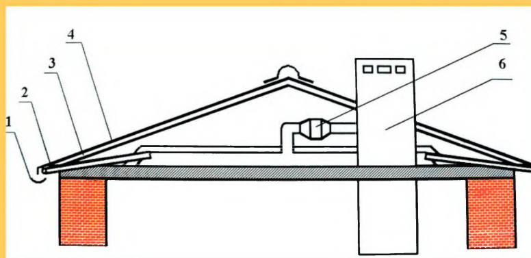
Схема подогрева воды в водостоках отработанным теплом: 1 — жёлоб; 2 — воздуховод; 3 — стропила; 4 — кровля; 5 — вентилятор; 6 — солнечная батарея
