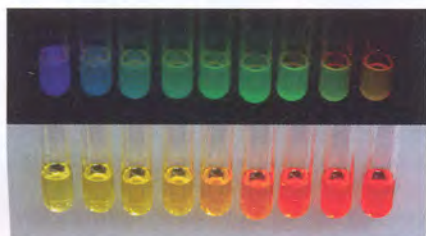
Рис. 4. Наночастицы CdSe в растворе. Размер частиц увеличивается слева направо от 2 до 12 нм. Вверху: в ультрафиолетовых лучах. Внизу: при дневном свете
