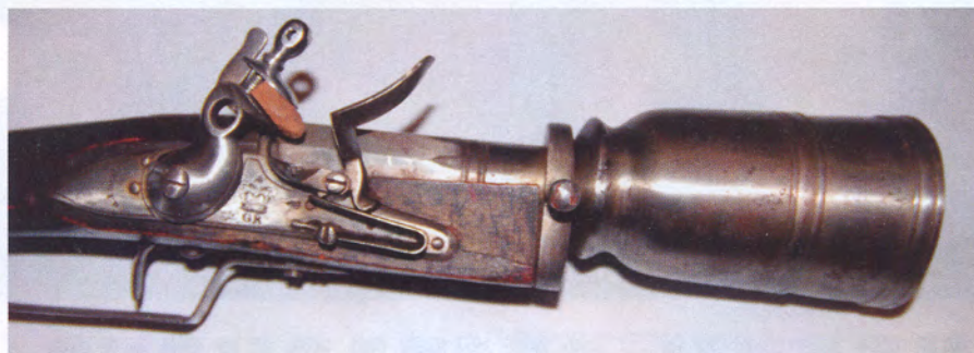
Ударно-кремнёвый замок и ствол драгунской мортирки
