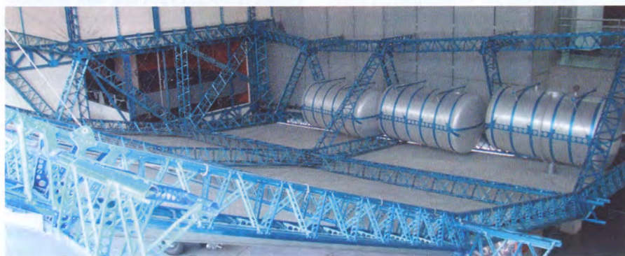
Реконструкция внутреннего устройства LZ 129 с баллонами для водорода
