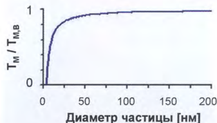
Рис. 7. Температура плавления золотых наночастиц в зависимости от их размера, отнесённая к температуре плавления «макрозолота»
