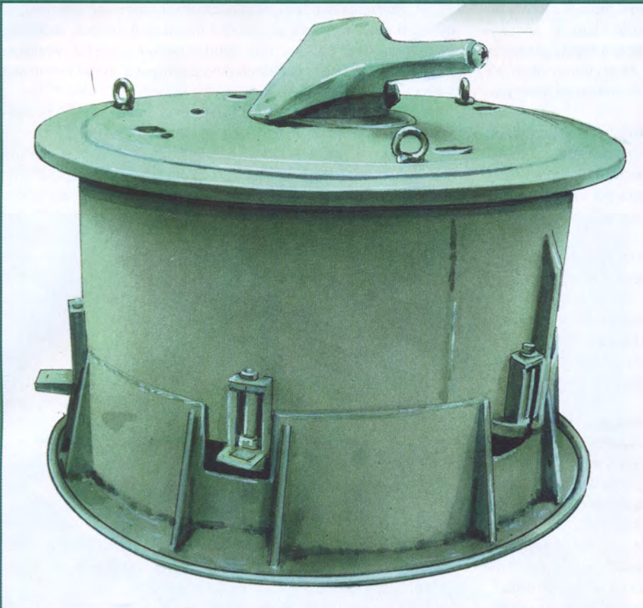
▲ Экспериментальный автономный модуль с кривоствольным пулемётом. СССР
