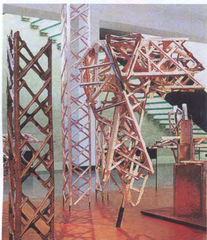
Дюралюминиевые узлы и опоры LZ 127, построенного в 1928 г.
