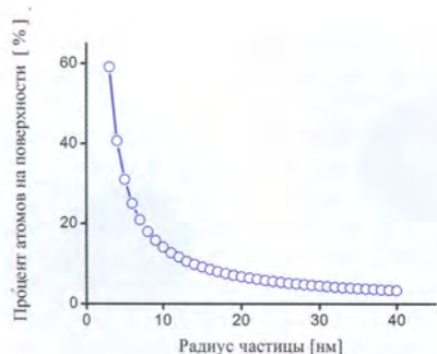
Рис. 1. Процент атомов на поверхности сферической частицы кобальта в зависимости от размера самой частицы
