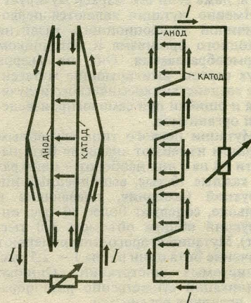
Рис. 2. Схема электрогенерирующего канала «Топаза-1» (справа) и «Топаза-2».
