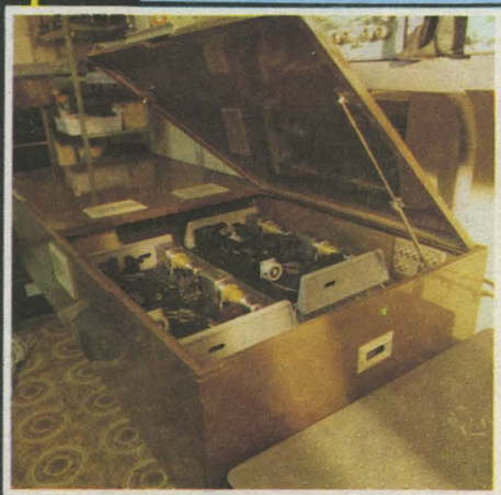
КАРС — спектрометр, созданный в виде прибора, достаточно компактен. Одна из его крышек приподнята, внутри видны лазеры.
