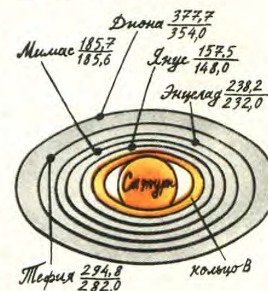
Сатурн с самым ярким кольцом В и пятью ближайшими спутниками. Верхние числа у спутников — истинные расстояния в тыс. км от них до центра Сатурна, нижние — определенные по формуле Г. Н. Левченко.
