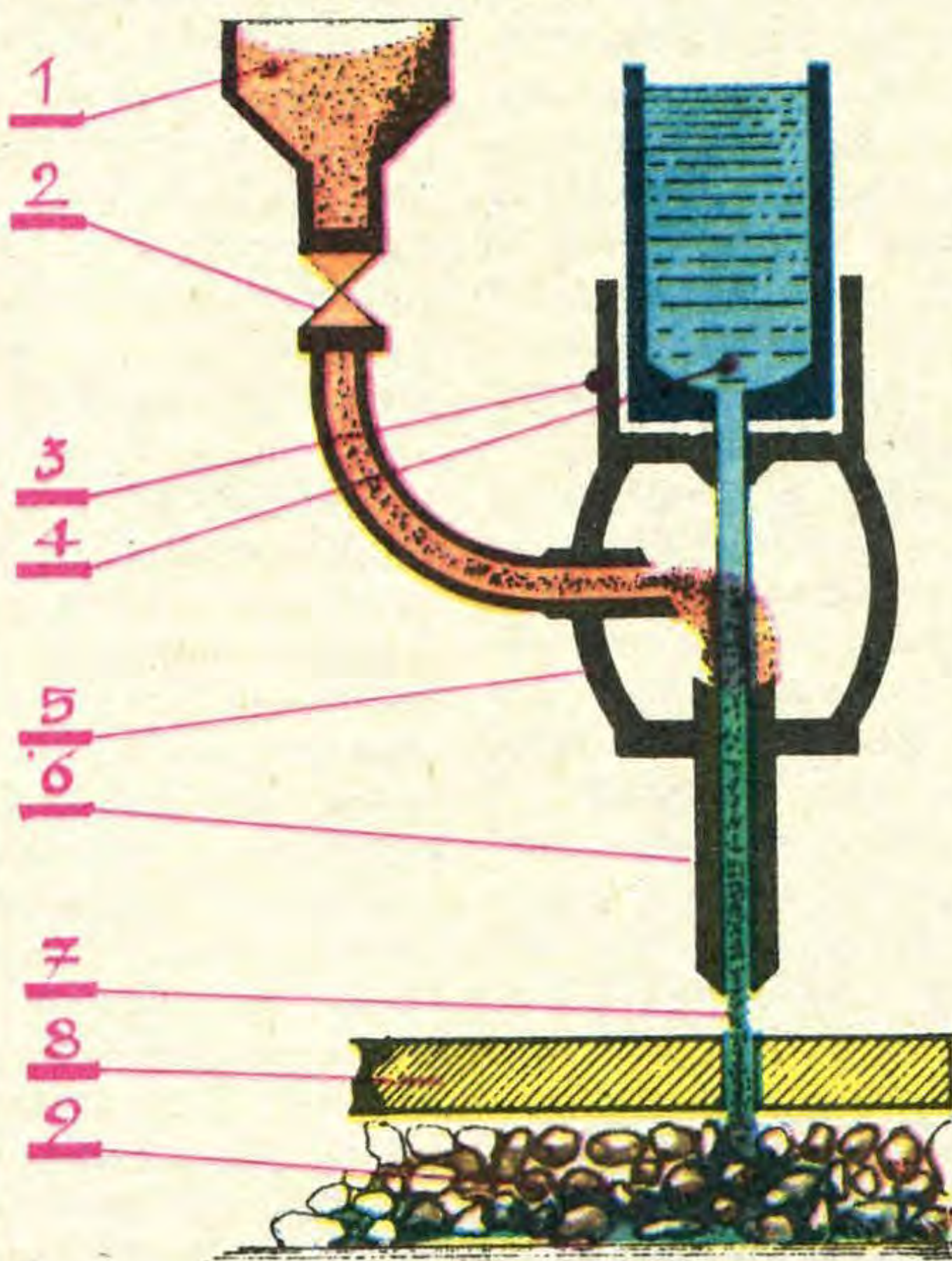
Принципиальная схема пазера.
