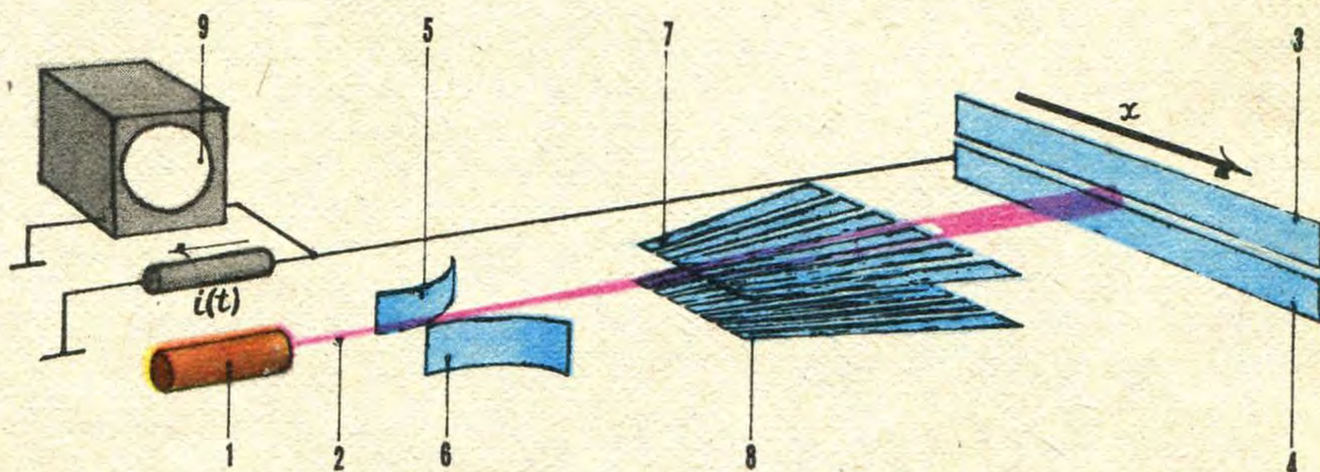
По внешнему виду политрон напоминает радиолампу. На снимке (с руками) — он же, только в металлическом кожухе. На схеме — устройство политрона: электронная пушка (1), комплекты пластин — анодных (3 и 4), управляющих (5 и 6) и функциональных (7 и 8), осциллограф (9).
