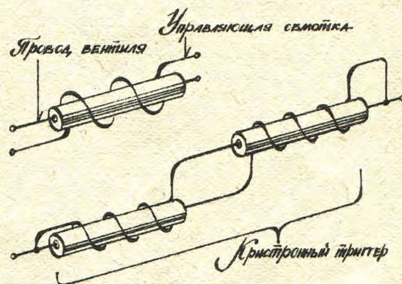
Р и с. 1. Проволочный криотрон.
