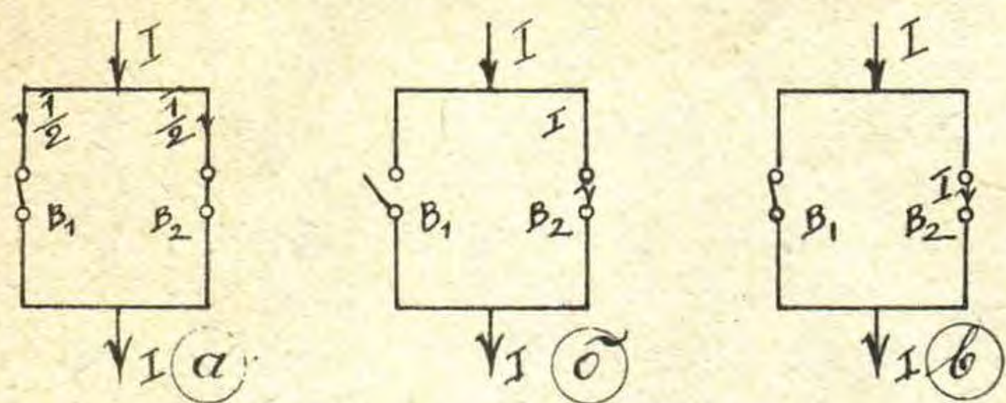
Р и с. 3. Принцип распределения сверхпроводящих токов.
