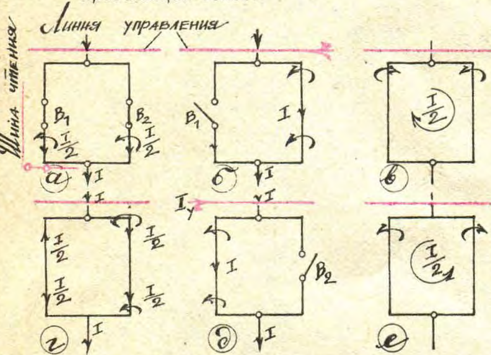
Р и с. 3. Принцип распределения сверхпроводящих токов.
