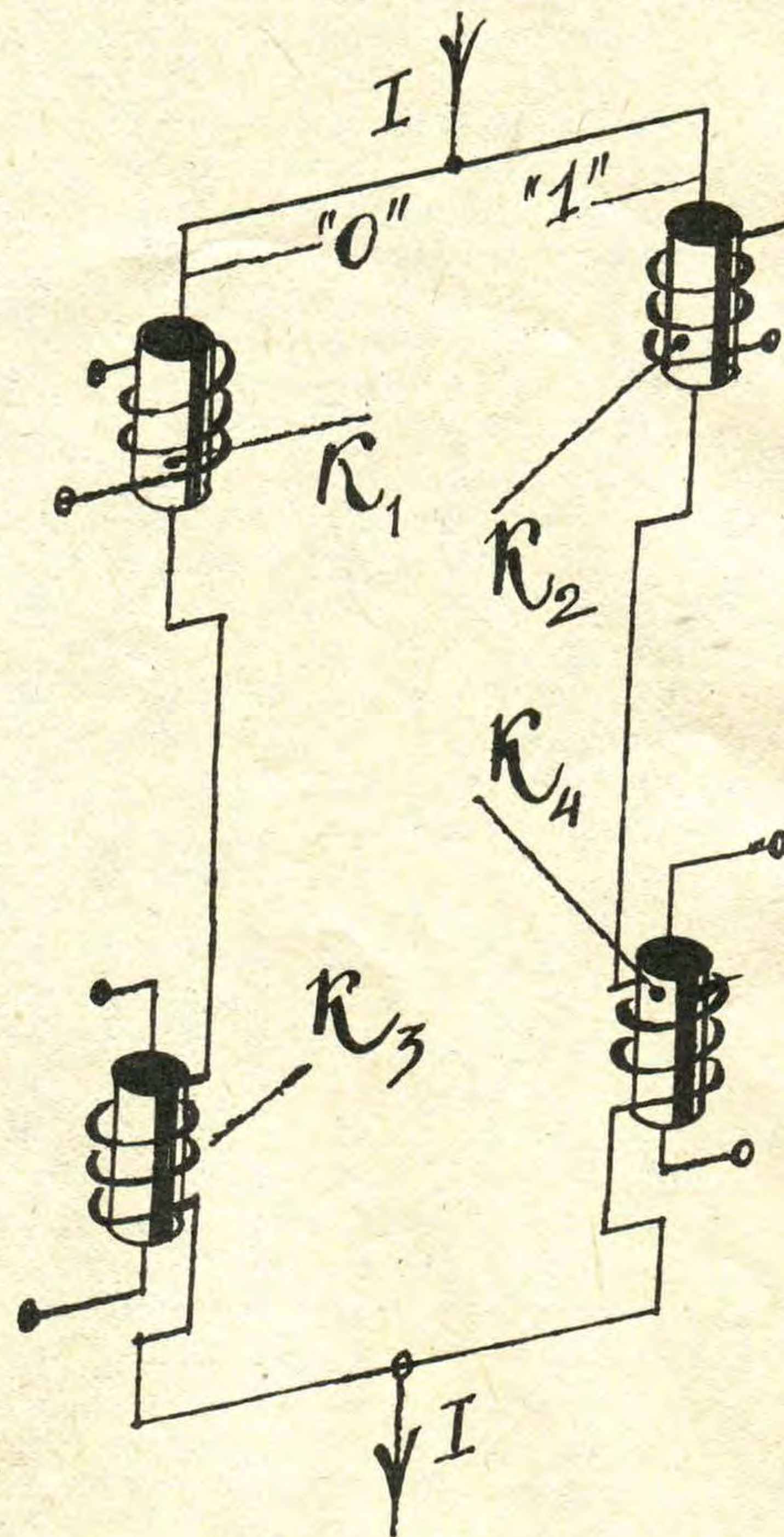
Р и с. 5. Схема коммутации на криотронах.
