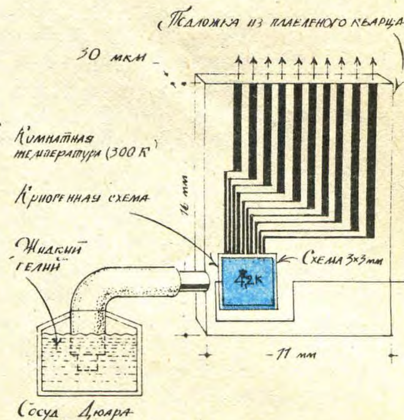
Рис. 9. Принцип открытого охлаждения.
