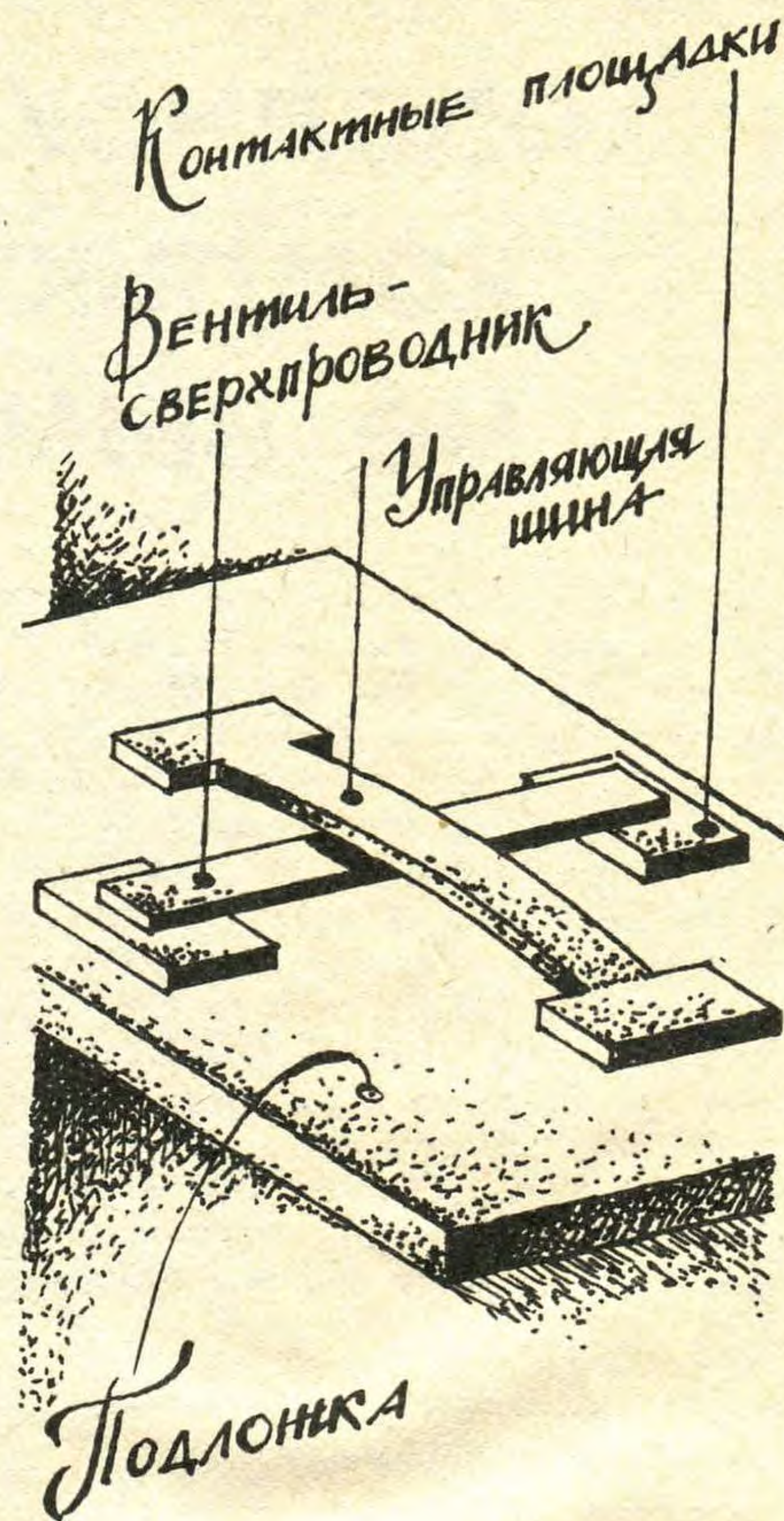
Р и с. 6. Пленочный криотрон.
