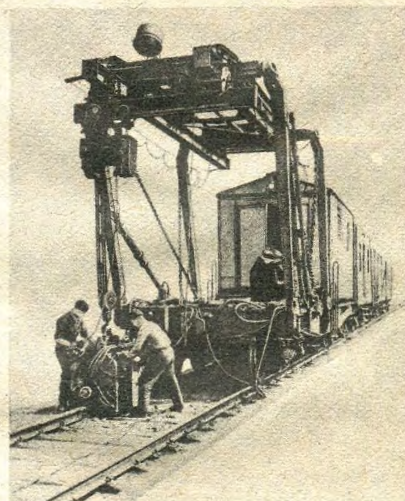
«Рельсосварочные машины ПРСМ? Но нам Минтяжмаш поставляет их так мало, что погоды они не делают», — сетует В. М. Бугаенко.
