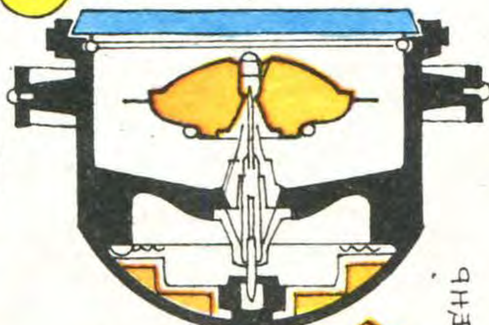
Котелок 75-мм магн. компаса
