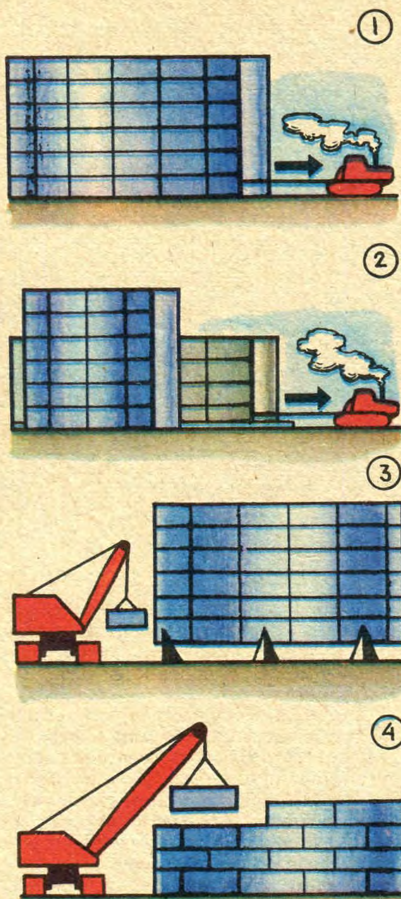
Варианты монтажа резервуаров емкостью 100 тыс. м 3 : 1) с однослойной стенкой из рулонов, 2) с двухслойной стенкой из рулонов, 3) с комбинированной сборкой, 4) с листовой сборкой.
