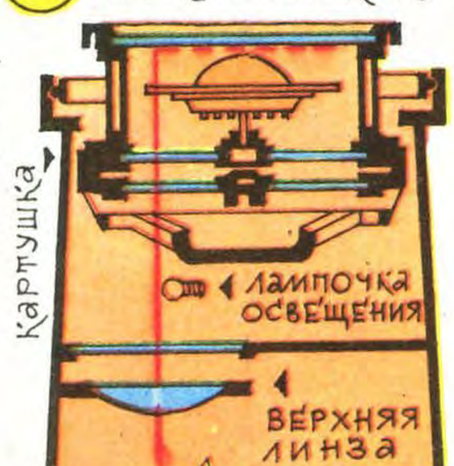
Оптическая система компаса "КМО-Т"
