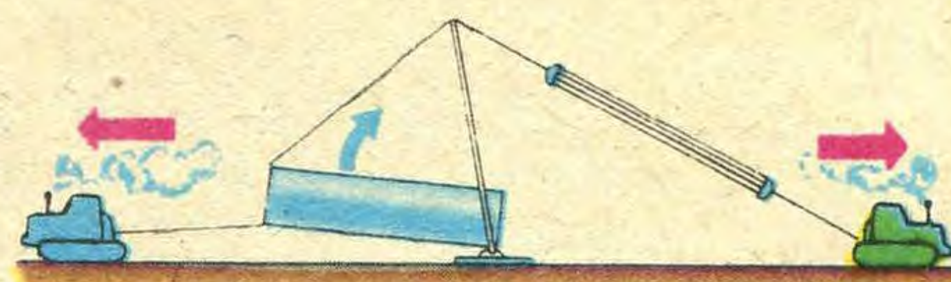
Подъем рулона с помощью «падающей» стрелы.
