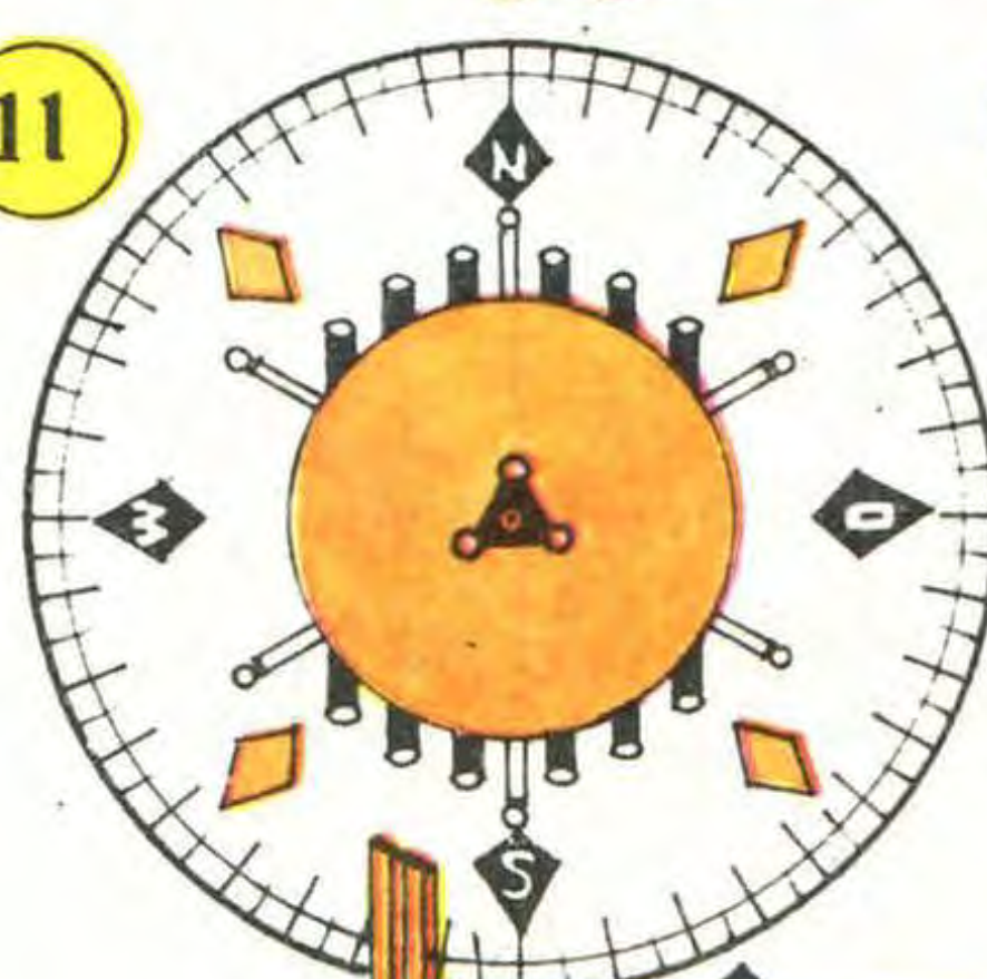
Картушка современного магнитного компаса Чашка дефлектора
