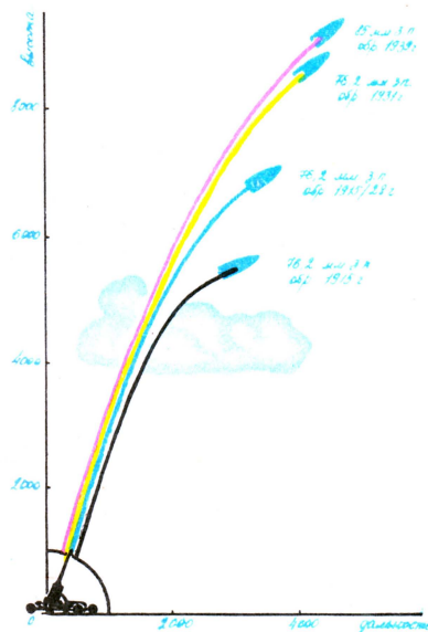
Траектории отечественных зенитных пушек (угол возвышения — 72°).
