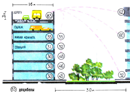
Распределение шума (в децибелах) от транспорта, движущегося по крыше здания.
