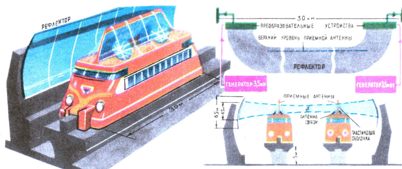
Аэропоезд с линейным электродвигателем, питающийся сверхвысоко-частотными радиоколебаниями. Справа — схема секции микро-волновой линии (вверху — вид сбоку, внизу — вид спереди).
