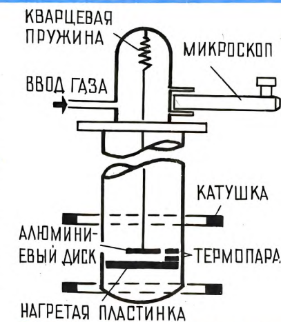
Газовые молекулы, разогнанные нагретой пластинкой, бомбардируют алюминиевый диск. Когда включается поле, добавляется терромагнитная сила.
