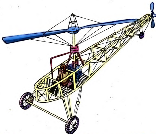
Проект Б. Юрьева — вертолет одновинтовой схемы с автоматом перекаса и рулевым винтом. Именно по такой схеме построено и строится в наши дни большинство винтокрылых машин.
