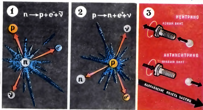
Реакции, порождающие нейтринно и антинейтринно.
