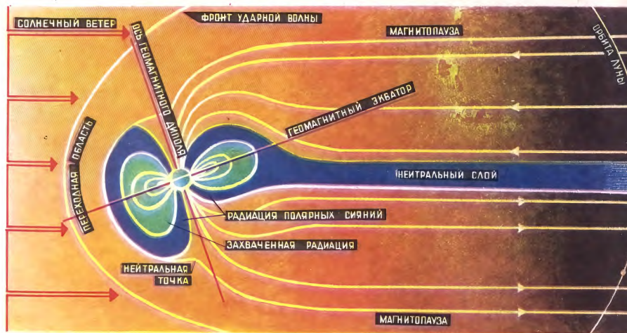
Искусственные спутники открыли сложную структуру околоземного пространства (магнитосферы).
