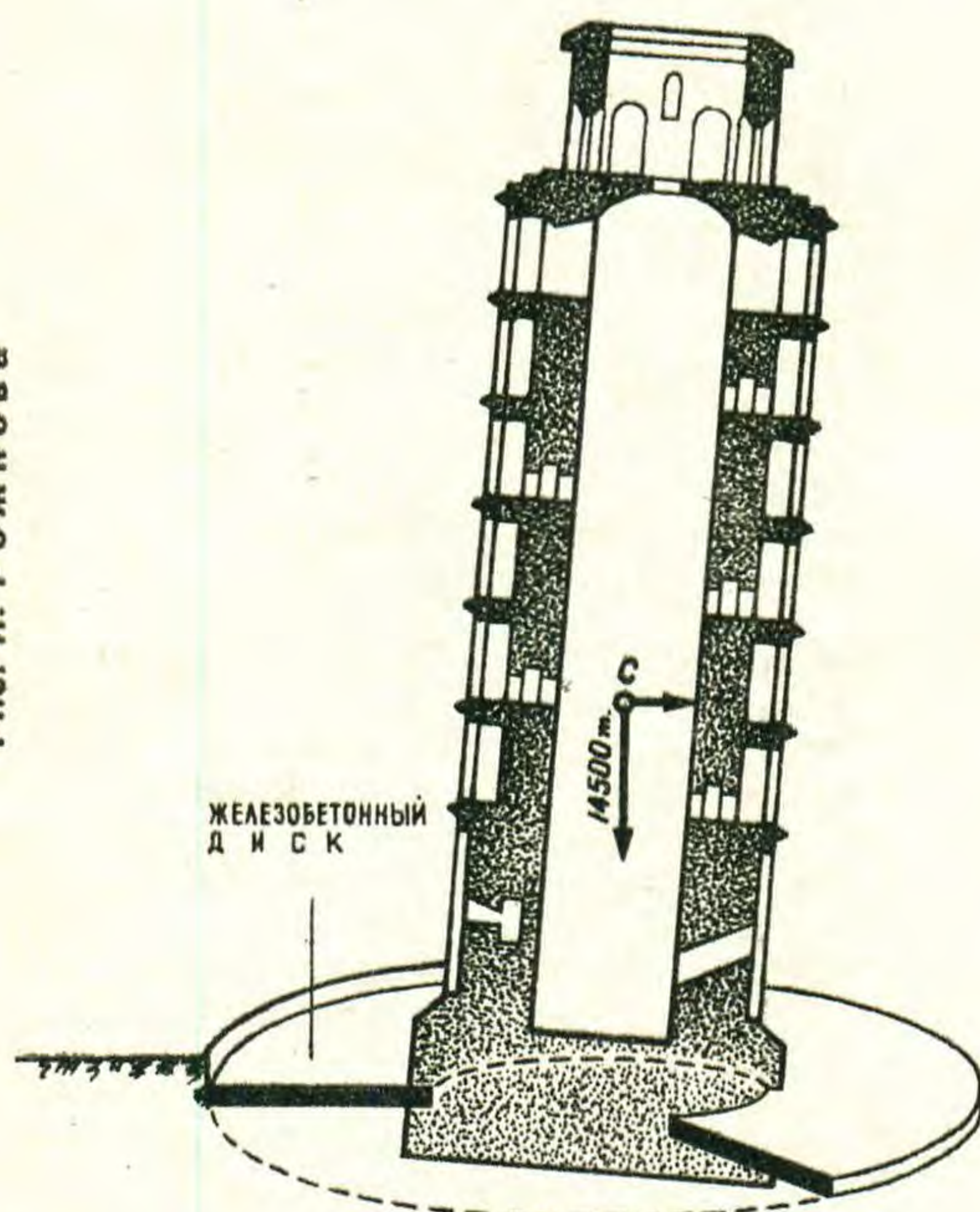
б) Вариант с жестким соединением башни и диска.
