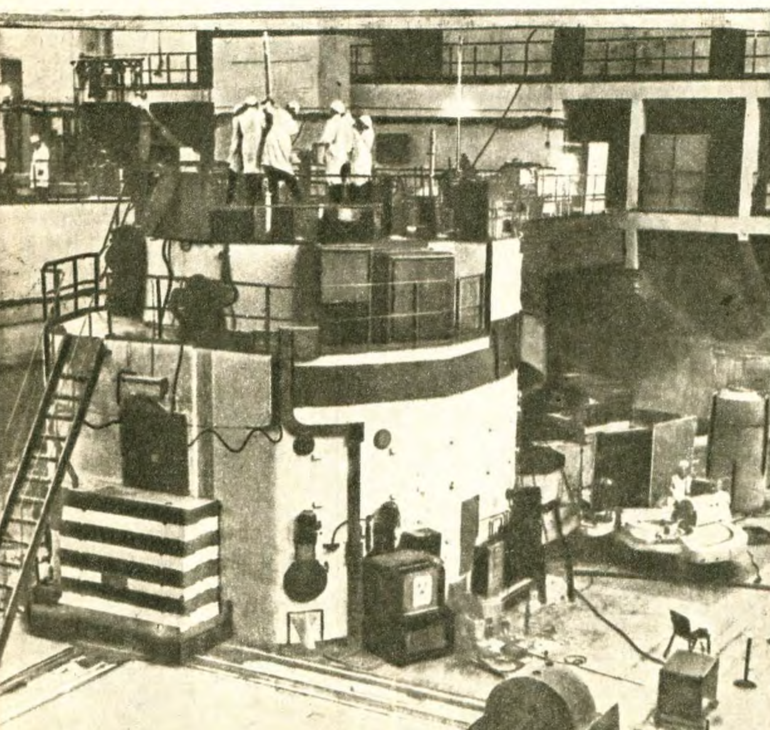
Самая совершенная техника исследования стала обычной в карповском институте в наши дни. На фото слева — исследовательский атомный реактор, справа — электронный микроскоп.
