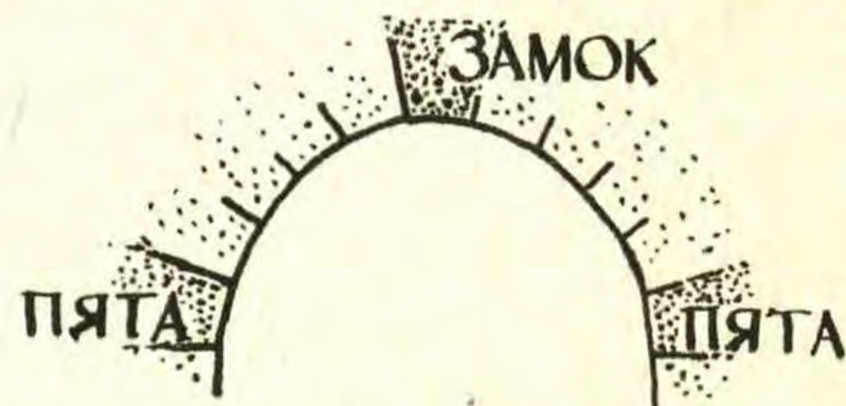
Кладка свода. Кирпичей нечетное число.
