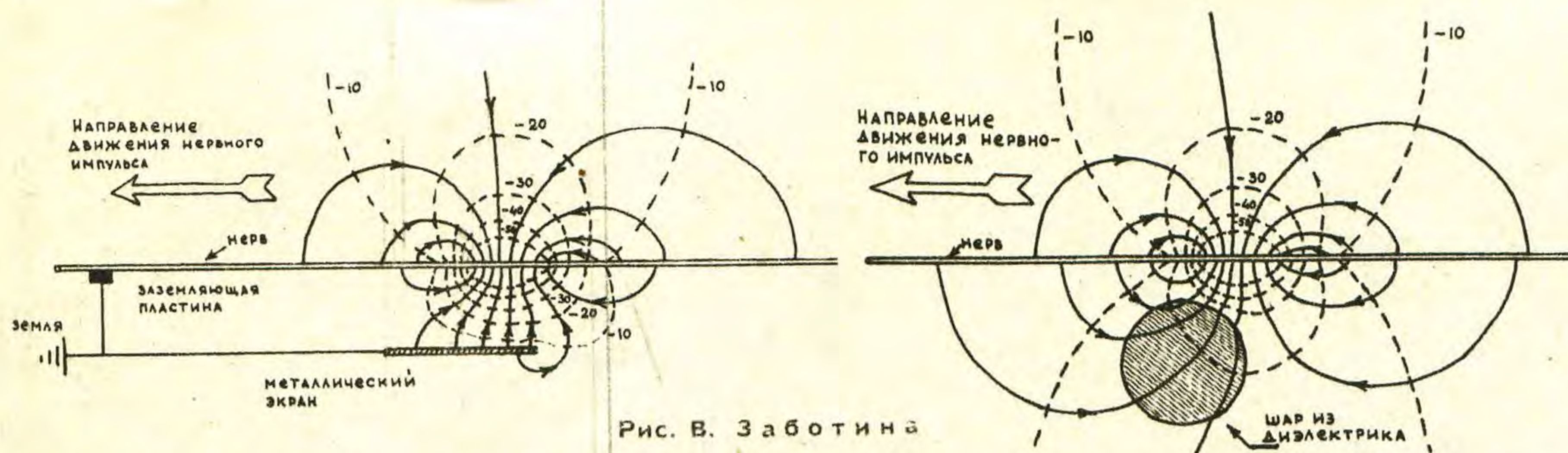
Рис. 1. Электрическое поле нерва искажается, если в пространство около нерва внести металлический экран или шар из диэлектрика. Пунктиром показаны изопотенциальные линии поля, то есть линии, по которым потенциал поля имеет одну и ту же величину (указанную в милливольтах). Силовые и изопотенциальные линии перпендикулярны друг к другу.
