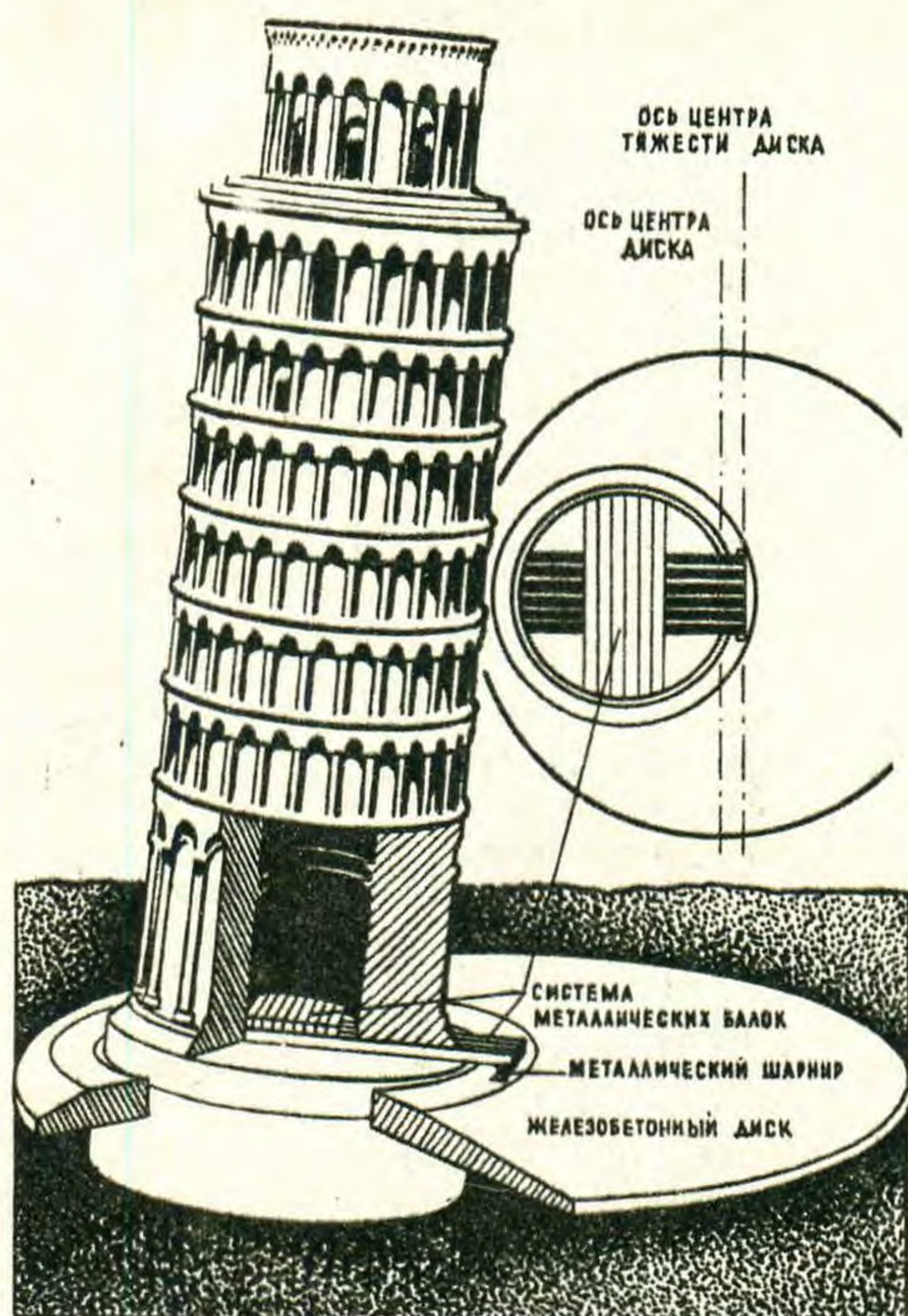
а) Вариант с шарнирным соединением башни и диска.
