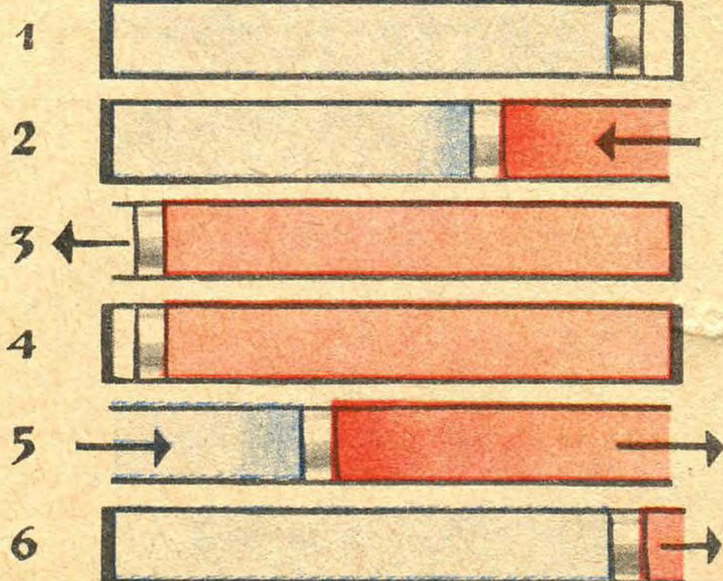
РАБОЧИЙ ЦИКЛ ПОРШНЕВОГО ГЕНЕРАТОРА
