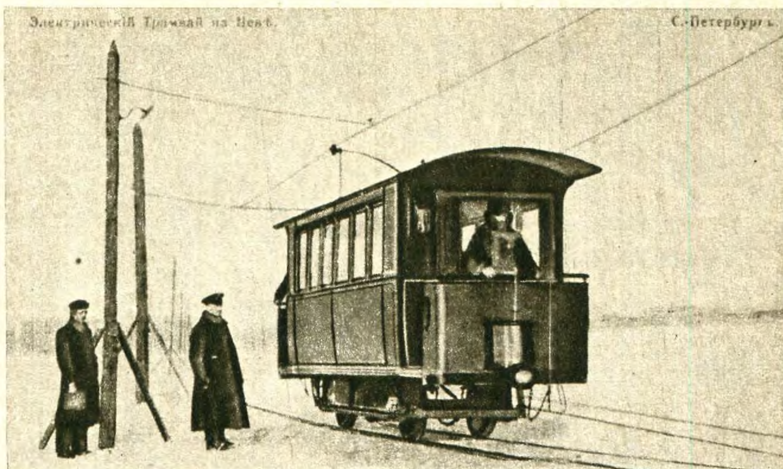
Электрический трамвай на Неве.
