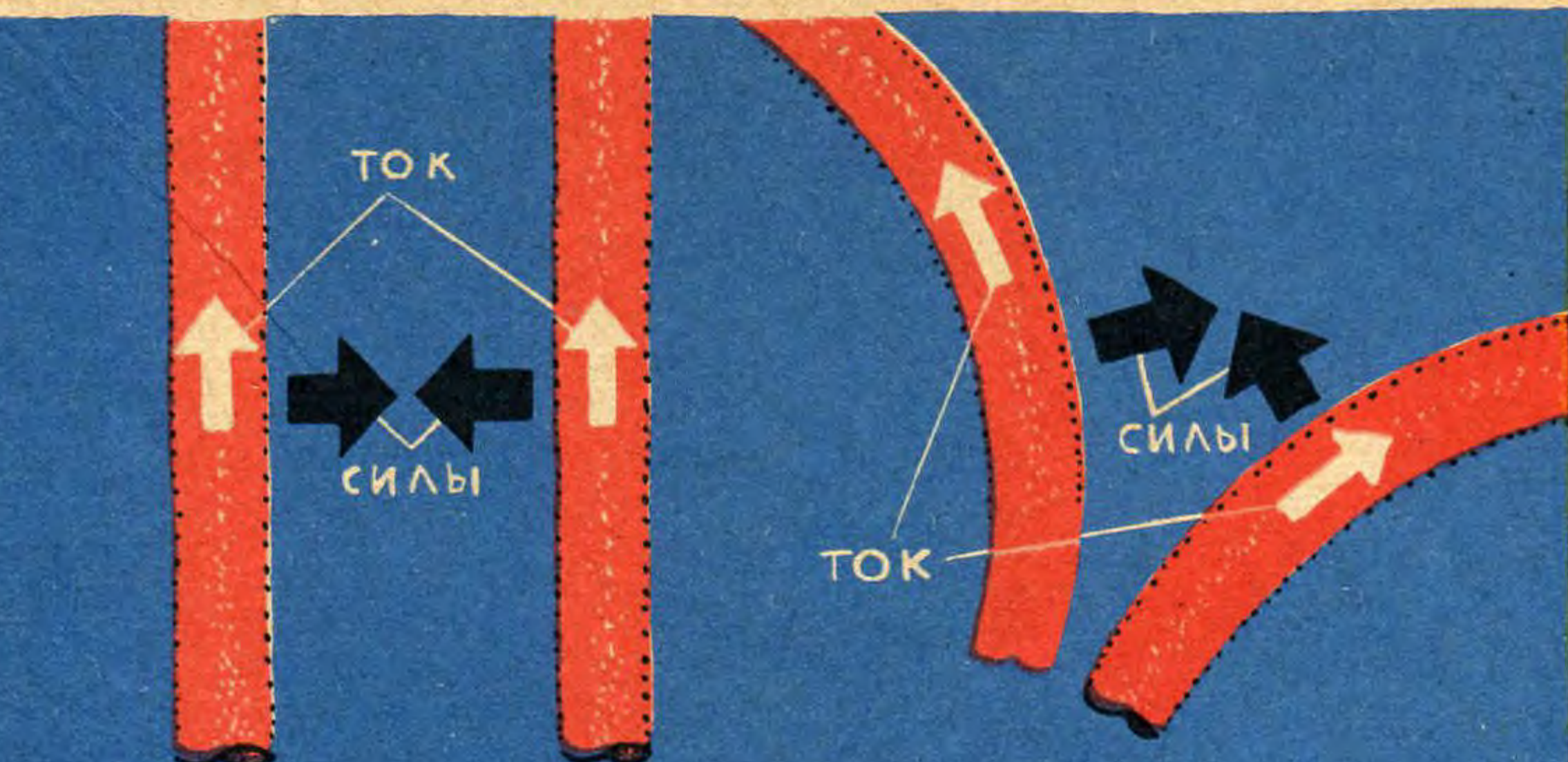
ВЗАИМОДЕЙСТВИЕ МЕЖДУ ЭЛЕМЕНТАМИ ТОКА ПО АМПЕРУ ПО ГРАССМАНУ
