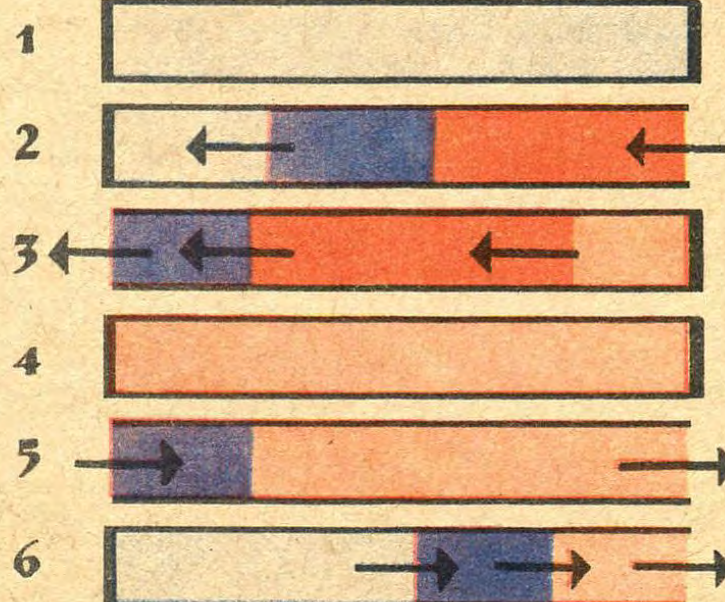
РАБОЧИЙ ЦИКЛ КОМПРЕКСА
