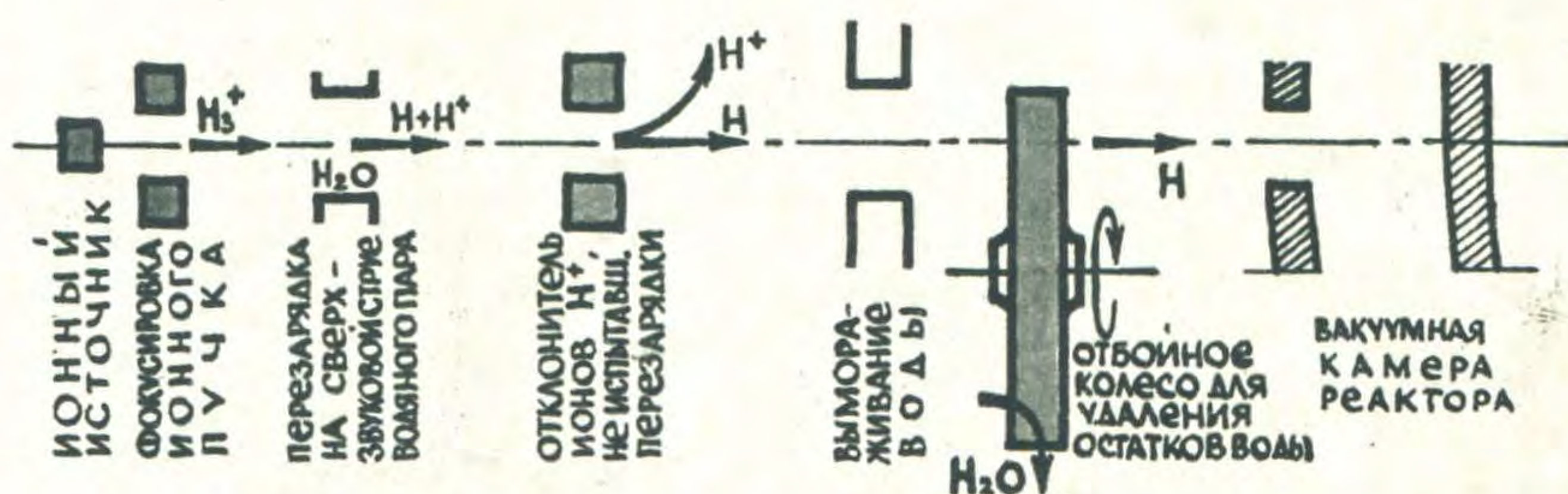
Схема инжекции нейтральных атомов водорода в вакуумную зону реактора.
