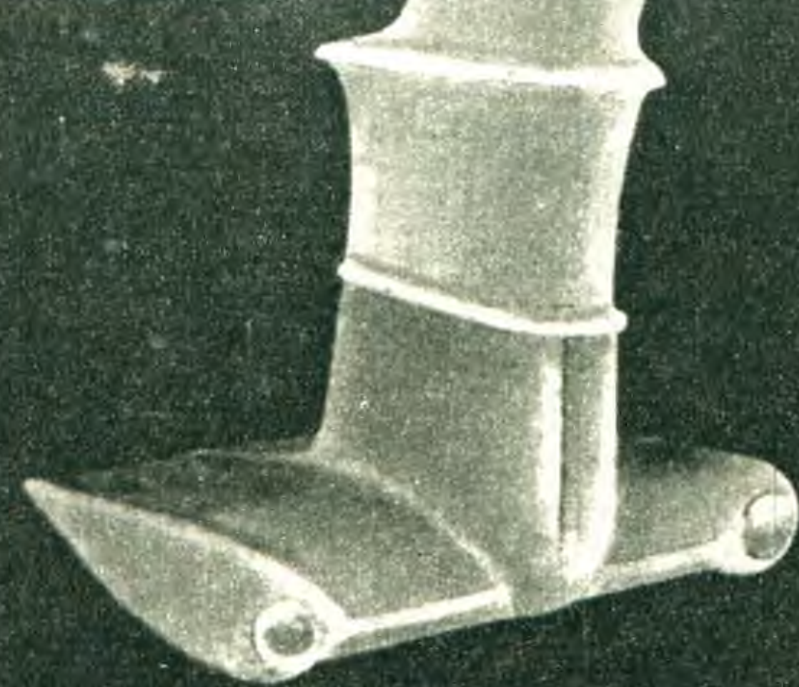
А так выглядит модель двигателя Коанда для современного судна на подводных крыльях.
