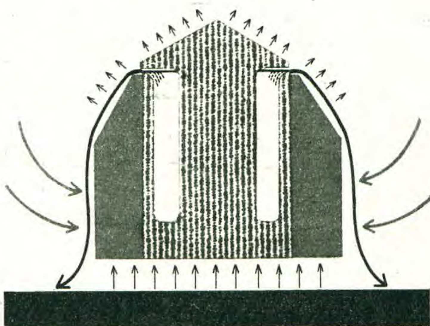
Схема действия внешнего сопла, работающего на эффекте Коанда. Поскольку давление под внешней поверхностью меньше атмосферного, а под днищем — больше его, такое сопло будет подниматься вверх.
